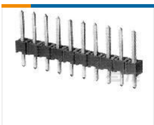
TE 零件编号826936-2 2P AMPMODU II STIFT LEI
