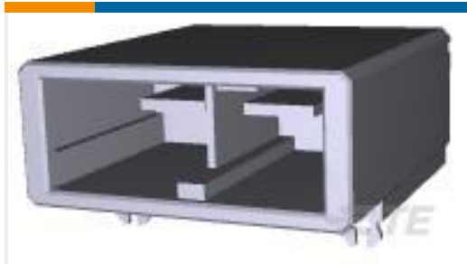
TE 零件编号1-353079-2 DYNAMIC D-5200 HDR H ASSY 2P
